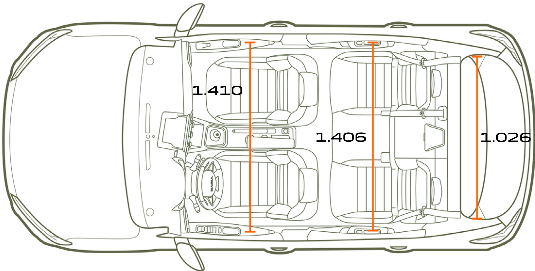
FRÅN OVAN
