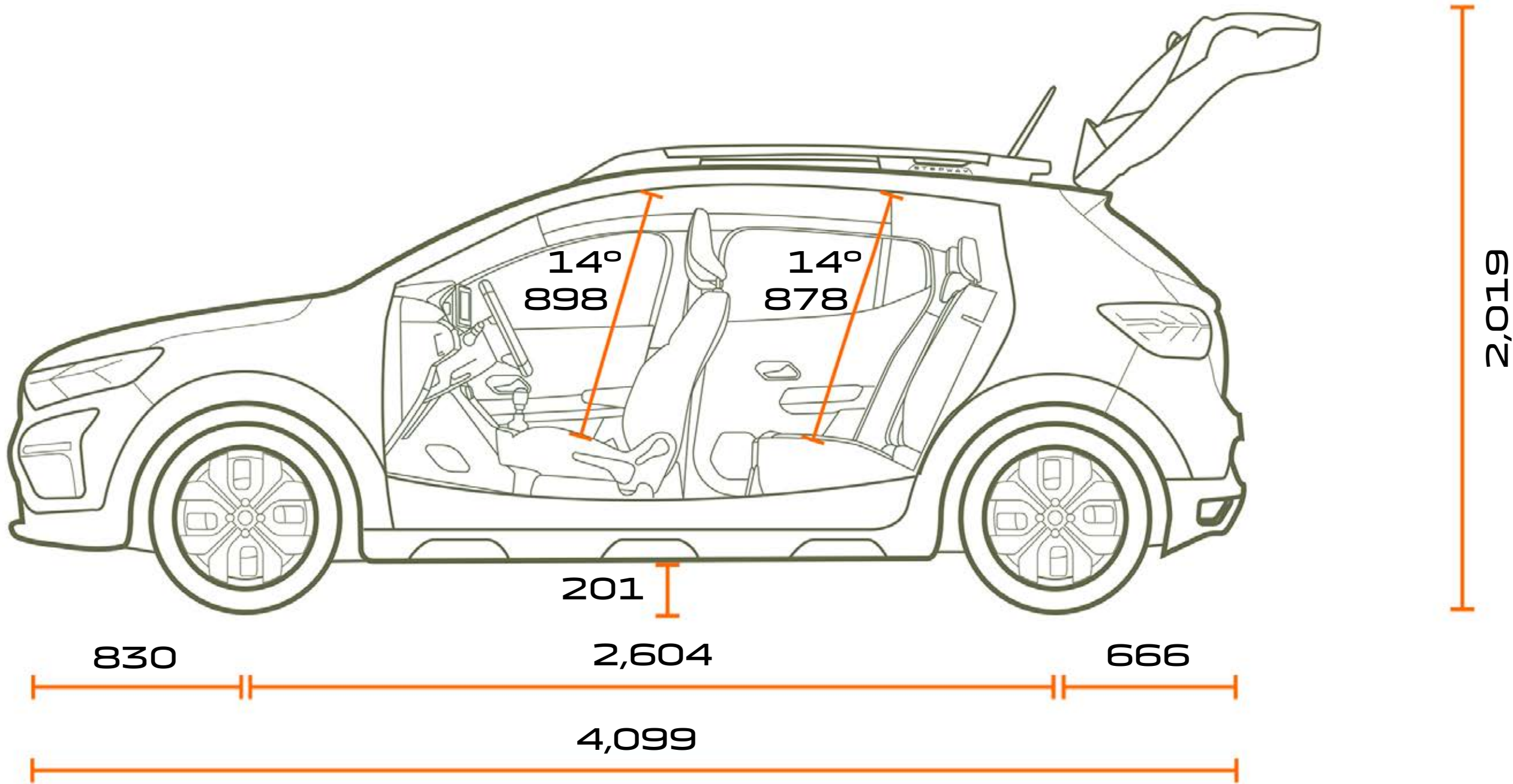
FRÅN SIDAN
